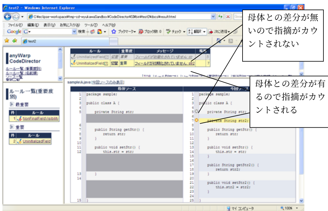
図. 母体ソースコードとの差分レポート出力画面
