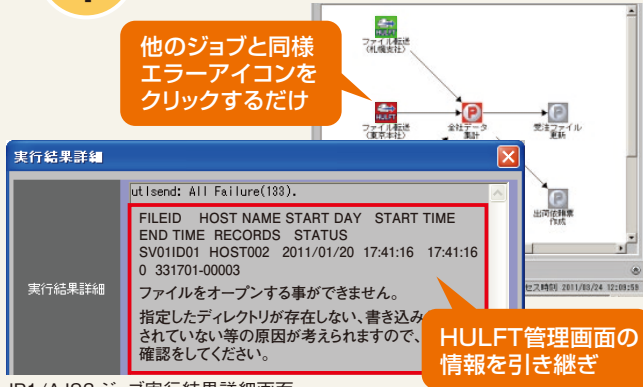
JP1/AJS3 ジョブ実行結果詳細画面
