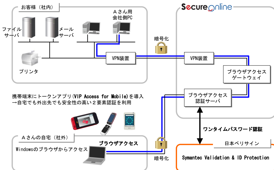
図. 2要素認証を利用した認証
