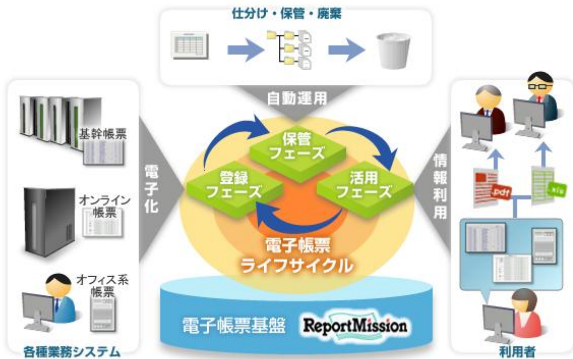
図.電子帳票基盤と電子帳票ライフサイクルの概要
