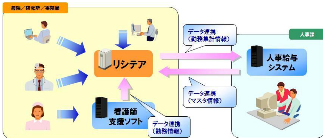
図. がん研究会のシステム構成
