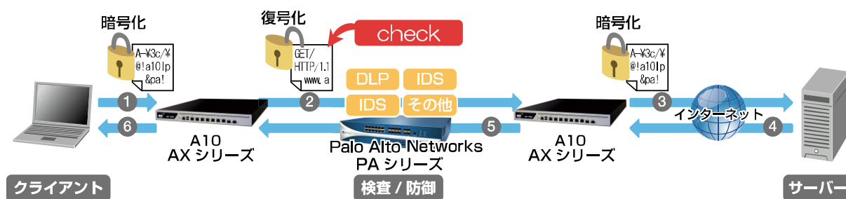
図:SSLインターセプト機能の概要
