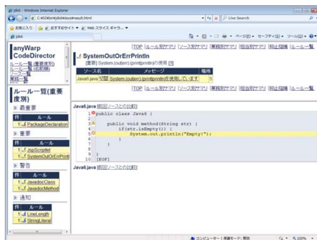
図1. JDK6.0, IE8 対応指摘画面例
